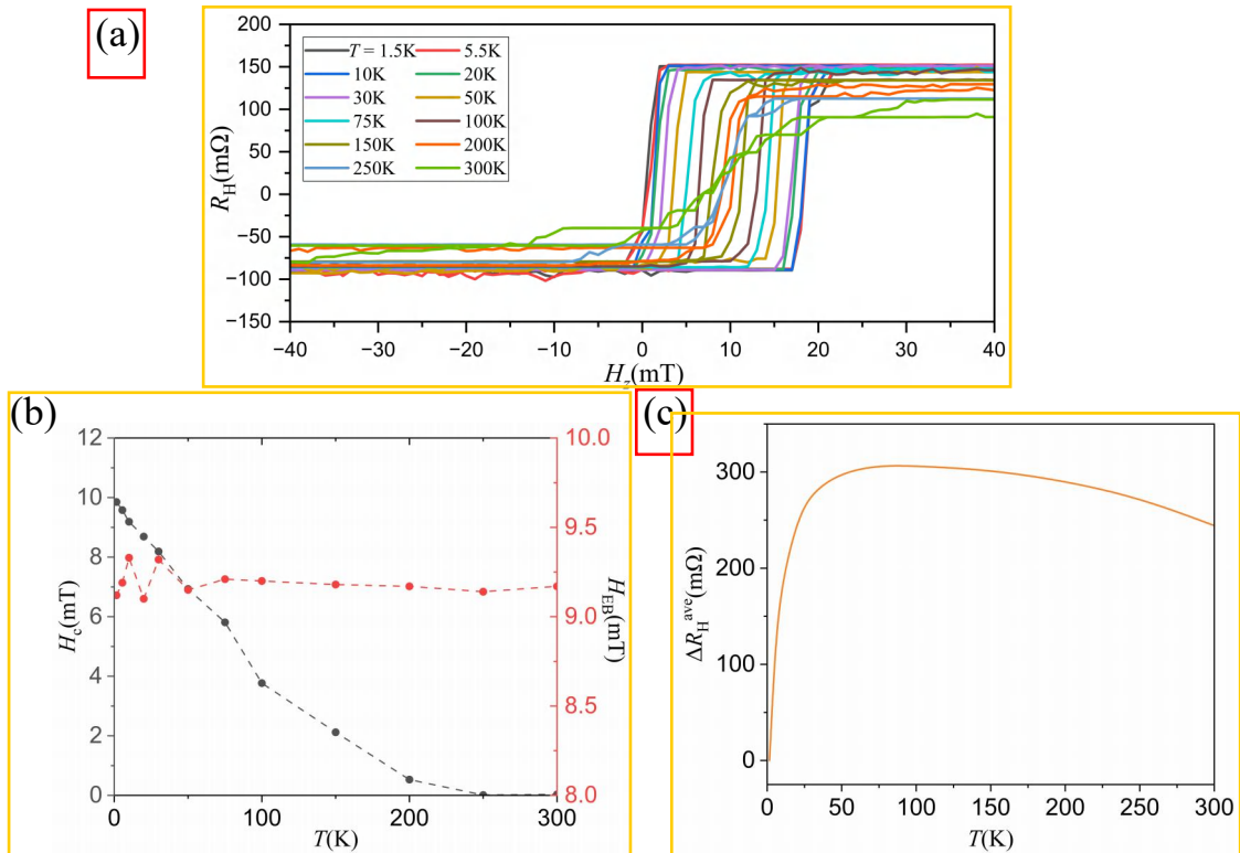
图 5.7 变温测试结果
