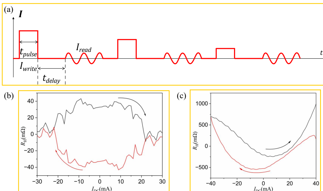
图 5.4 面外磁化器件的 SOT 翻转
