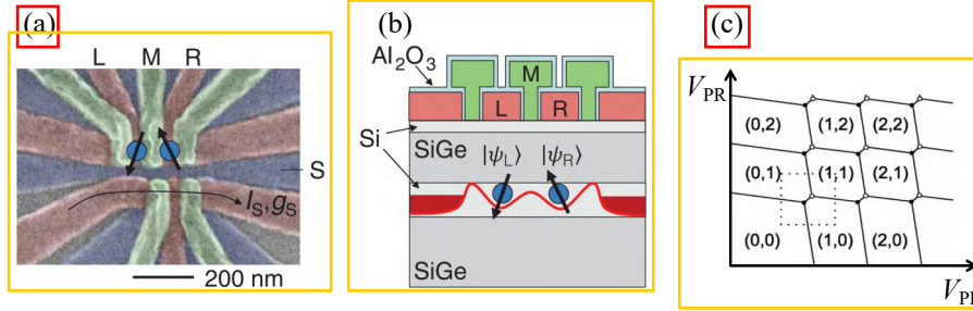
图 2.3 双量子点结构与电荷稳态分布图
