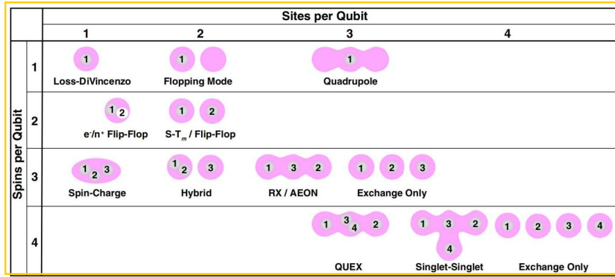
图 2.5 按每个量子比特所含自旋和量子点数量分类的各种自旋量子比特
