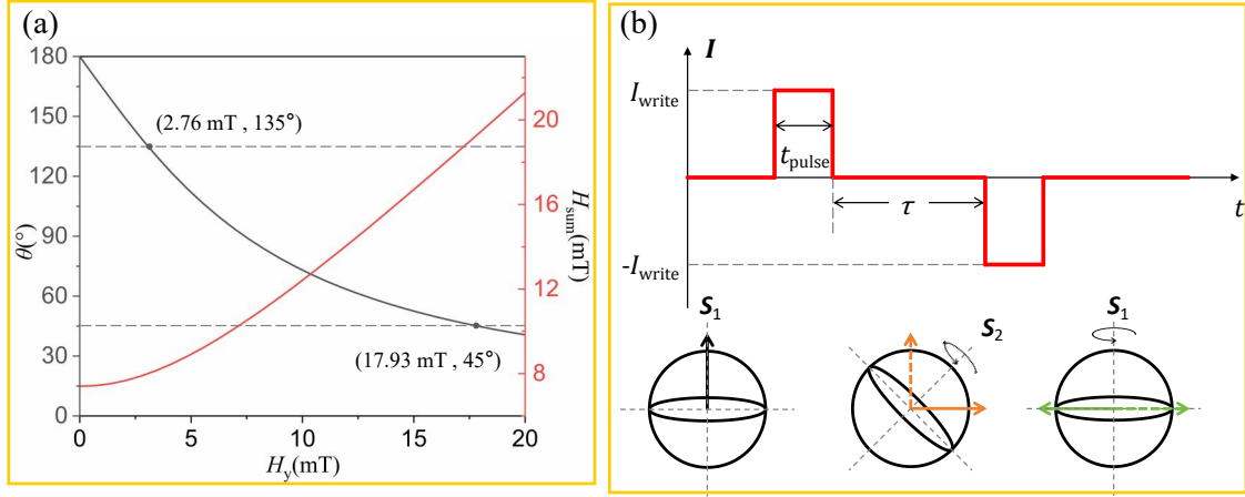
图 3.7 有外加辅助磁场的单面外磁化 SOT 器件的方案
