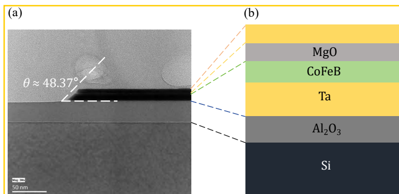
图 4.5 以面内构型为例展示制备的 SOT 器件剖面视图
