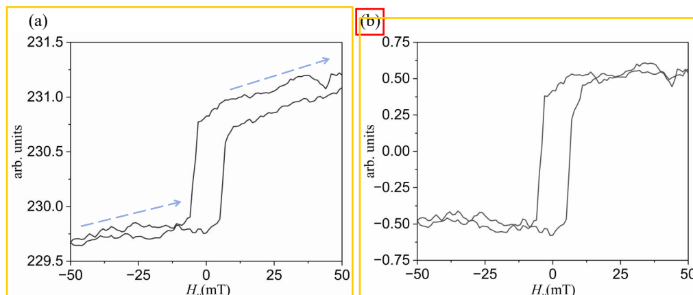
图 4.3 MOKE 测试结果及数据处理后的对比
