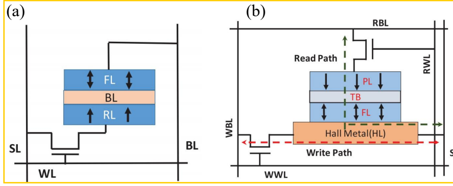
图 2.7 器件写入方式的对比
