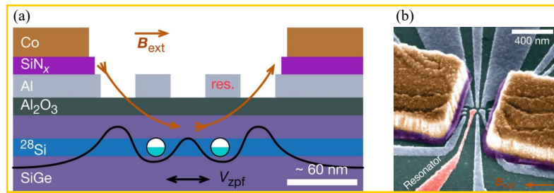
图 1.1 硅基量子器件中的微磁体
