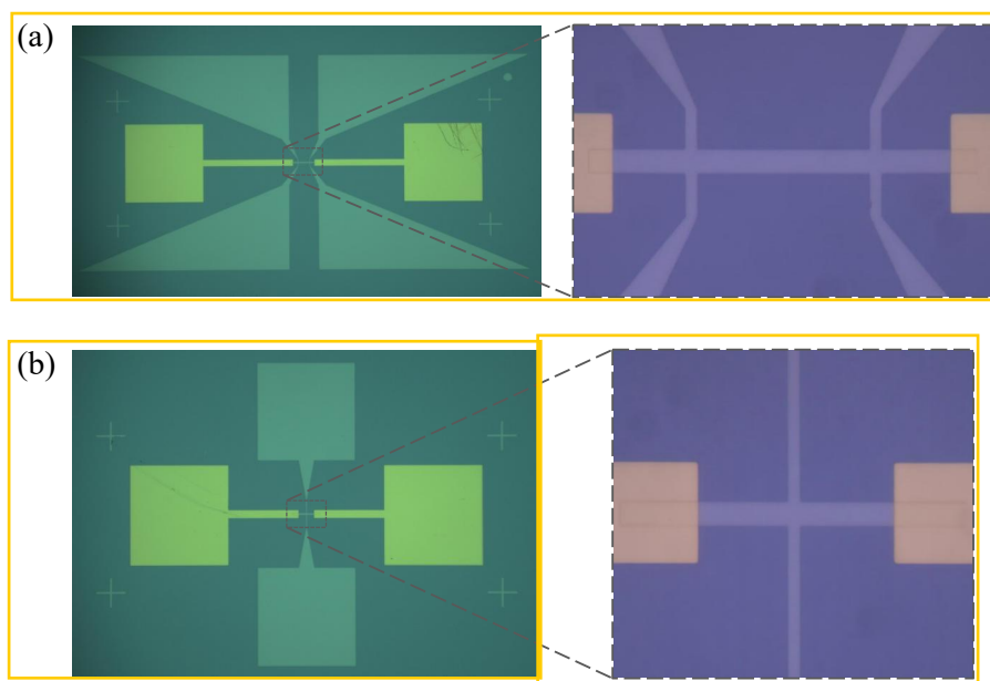
图 4.6 用于测试的 SOT 器件光学照片
